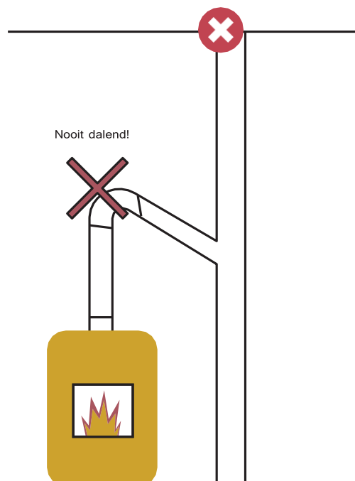
fig. 4 Het aansluitkanaal mag nooit in dalende lijn geplaatst worden.
