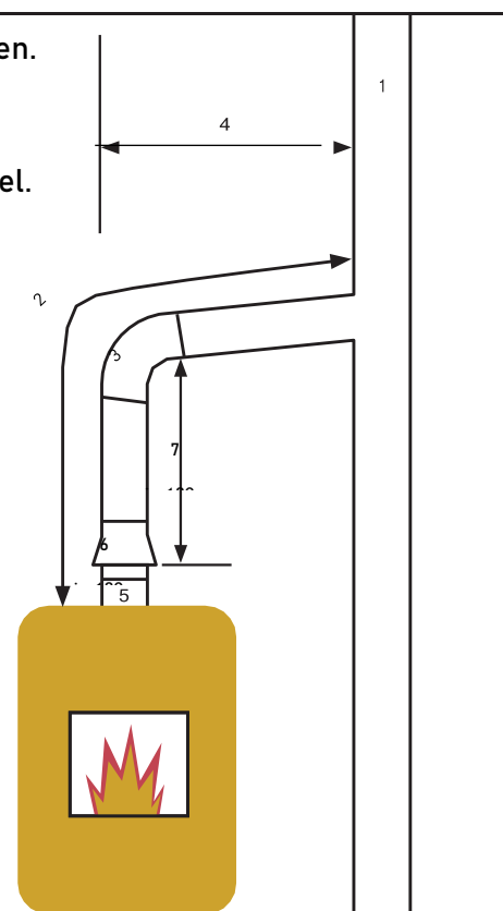
fig. 2 Voorbeeld toestel type B1x met externe trekonderbreker (onderdelen).
