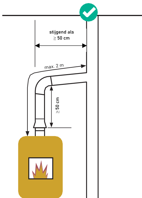
fig. 3 Voorbeeld toestel type B1x met externe trekonderbreker (afmetingen).
